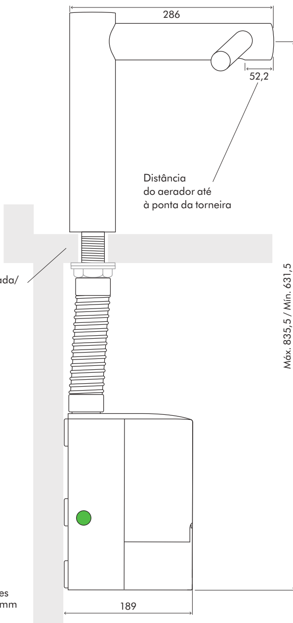
ELEVAÇÃO LATERAL
