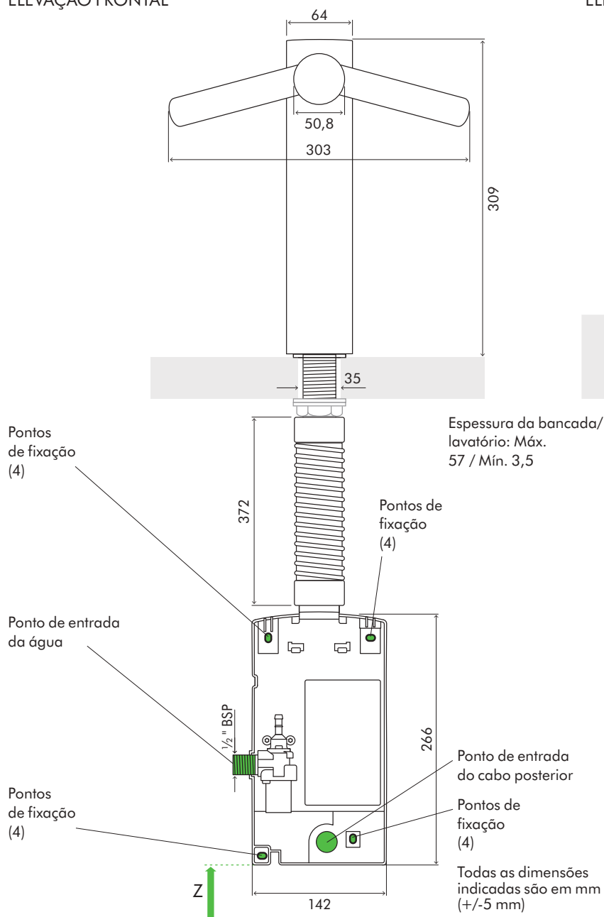
ELEVAÇÃO FRONTAL
