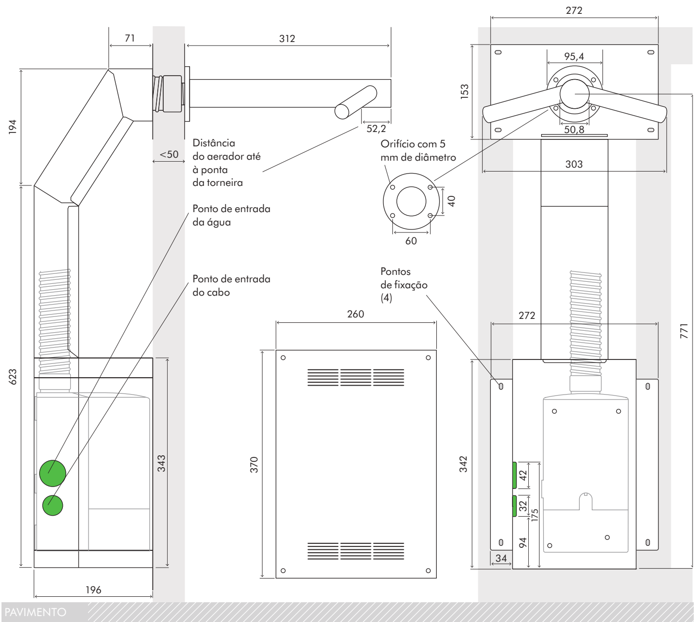
ELEVAÇÃO LATERAL
